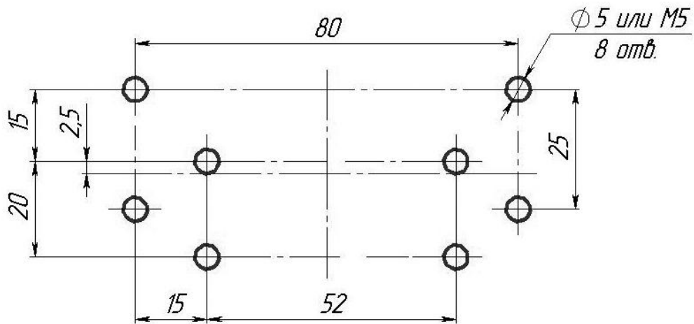
Разметка для крепления на щите
