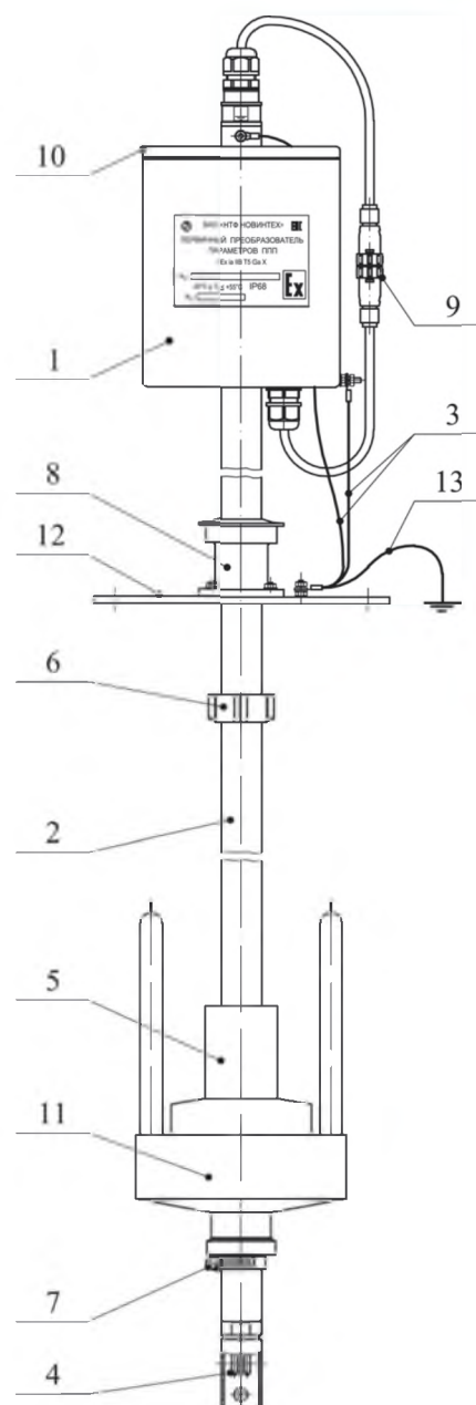
Рисунок 2 - ППП для АЗС с датчиками уровня, воды, температуры и плотности (поверхностный) с возможностью подключения ДД1, ДУТ
