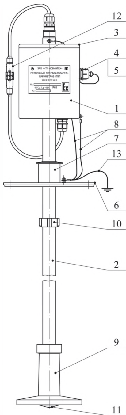
Рисунок 8 - ППП для градуировки резервуаров (ГР) с высотой залива до 4000 мм
