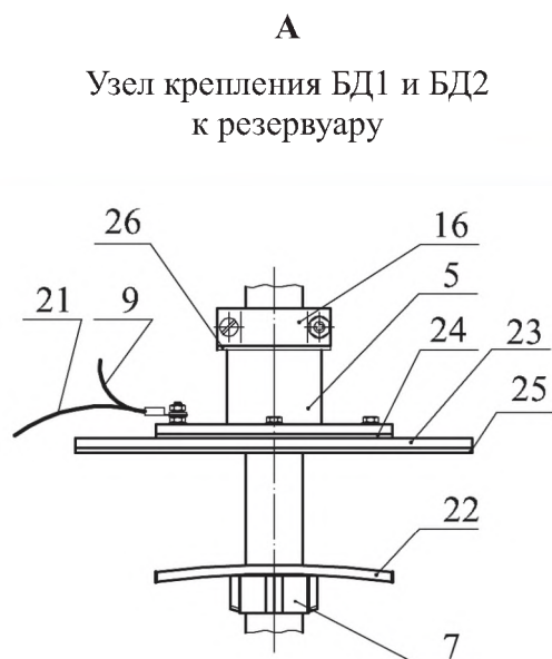
Рисунок 5 - ППП для НБ с датчиками уровня, воды, температуры, плотности (погружные) с установкой на два фланца
