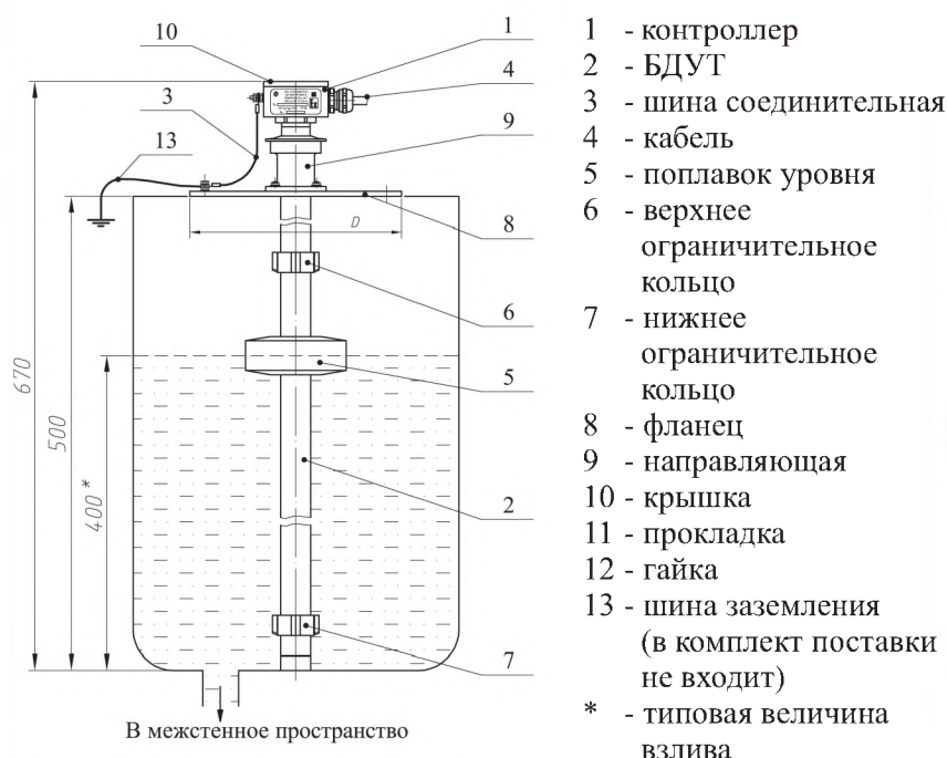
Рисунок 13 – ДУТ 306 с датчиками уровня и температуры
