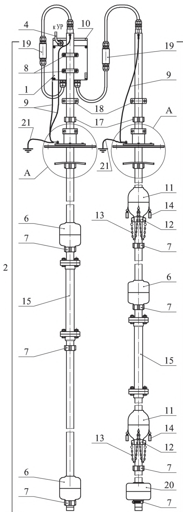
Рисунок 5 - ППП для НБ с датчиками уровня, воды, температуры, плотности (погружные) с установкой на два фланца
