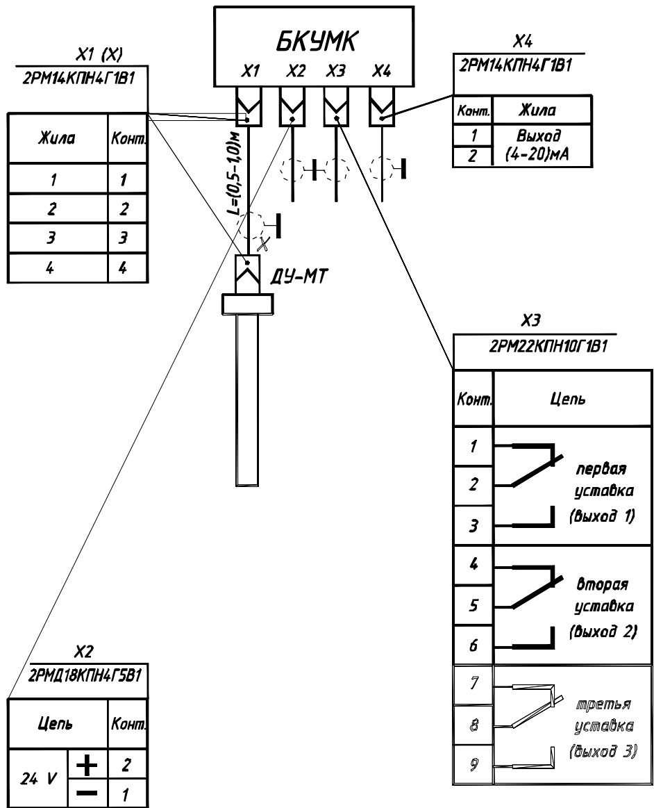
СХЕМА ВНЕШНИХ СОЕДИНЕНИЙ ПРИБОРОВ ПКУМК
