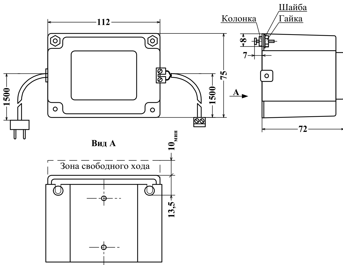
а) внешний вид ИЭП
