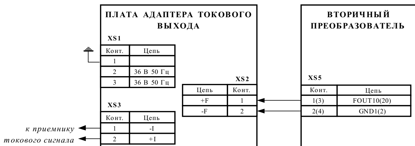
Рис. Г.2. Схема подключения платы адаптера.
