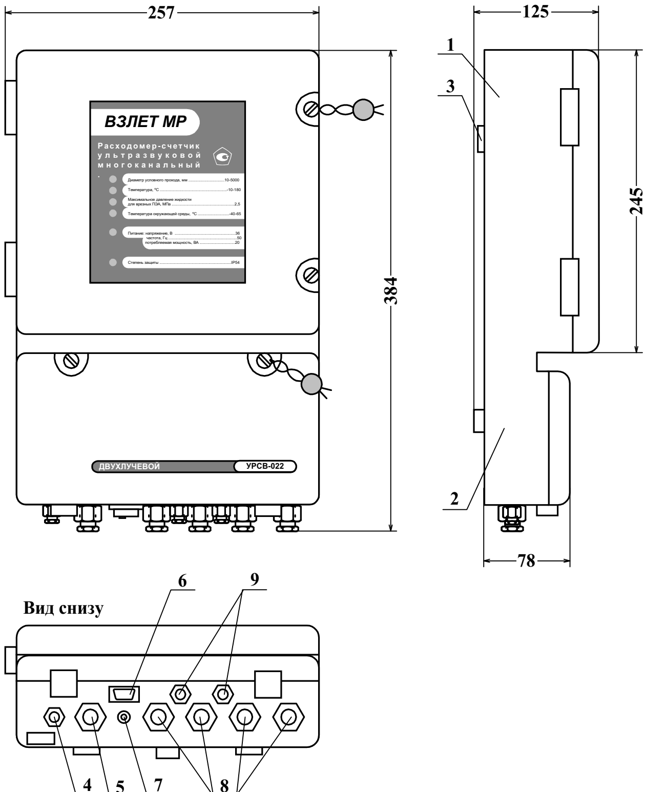
Рис. А.1. Внешний вид ВП.
