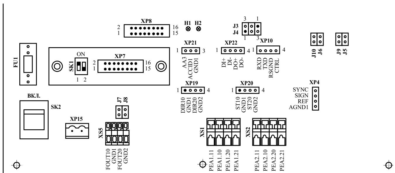
Рис. Б.2. Размещение элементов коммутации и управления на системной плате.
