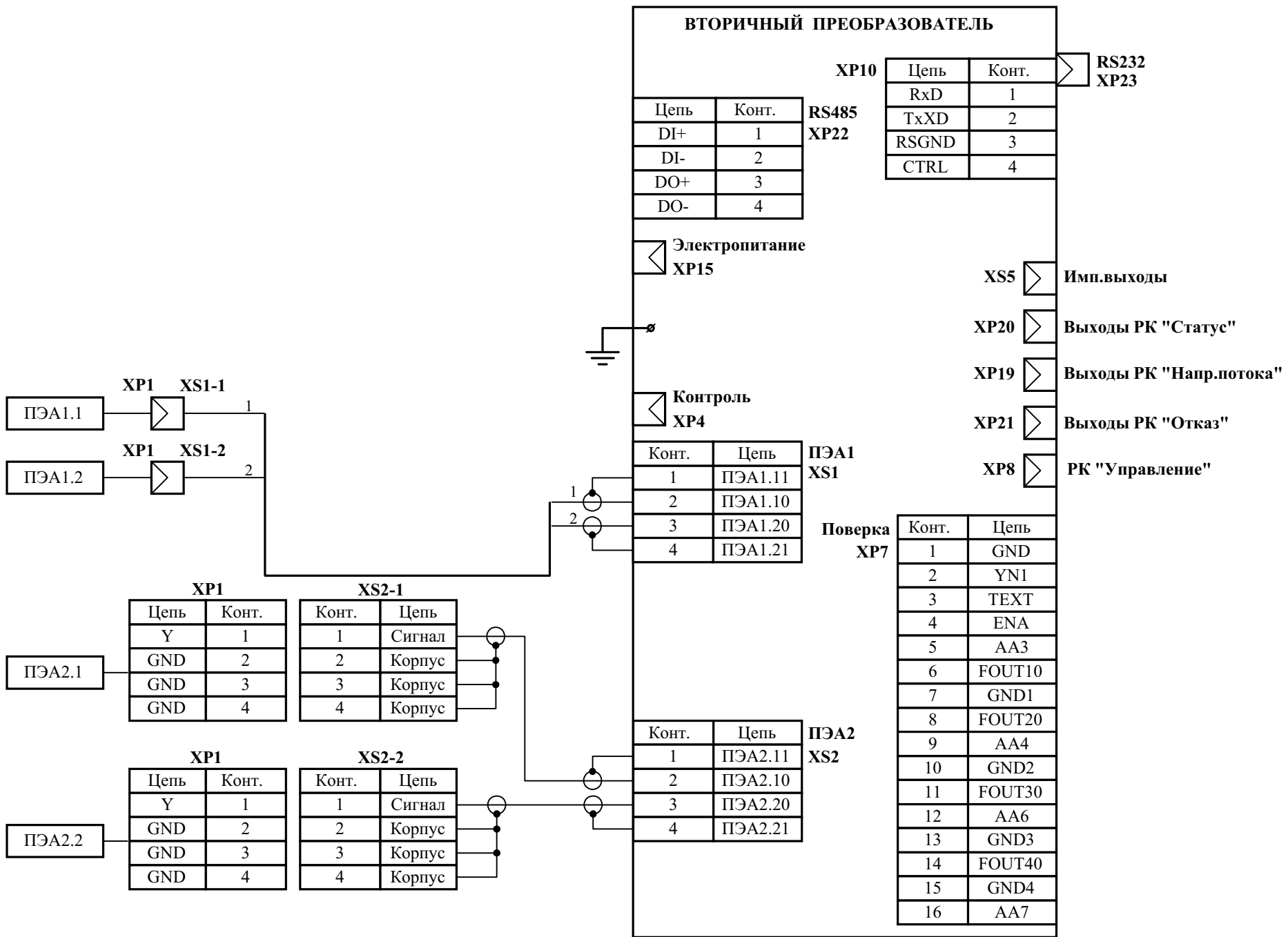
Рис. Б.1. Схема соединений расходомера «ВЗЛЕТ МР» исполнения УРСВ-022.
