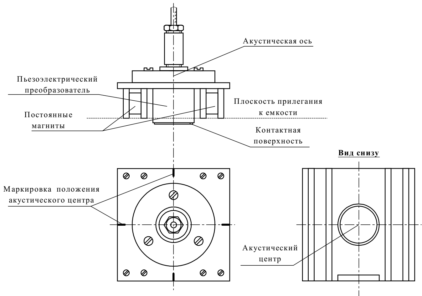
Рис. 3. Внешний вид датчика сигнализатора уровня.
