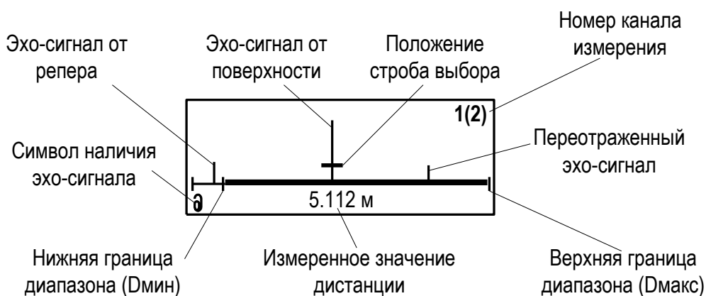
Рис.2. Вид окна Развертка.
