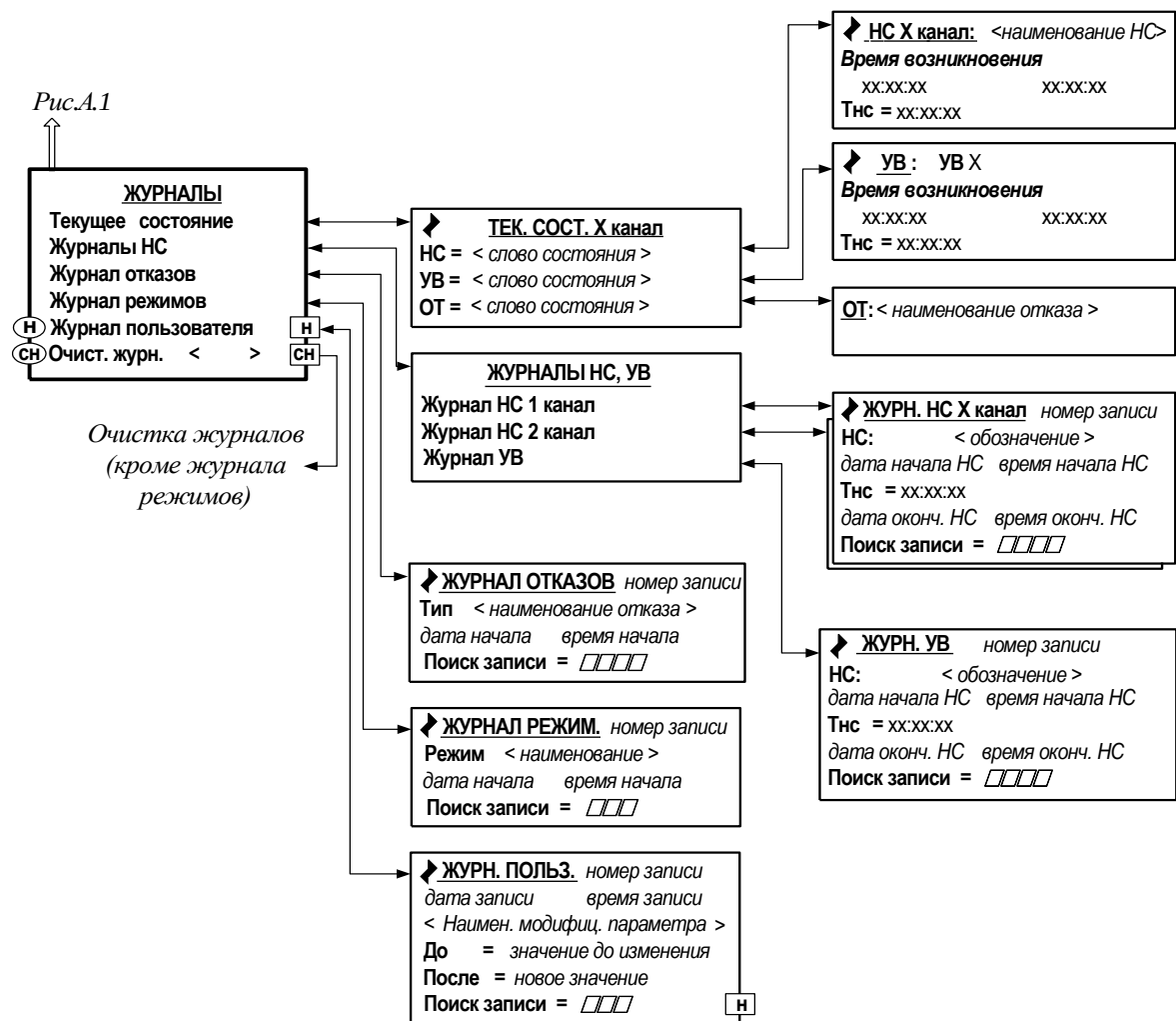
Рис.А.6. Меню «Журналы».
