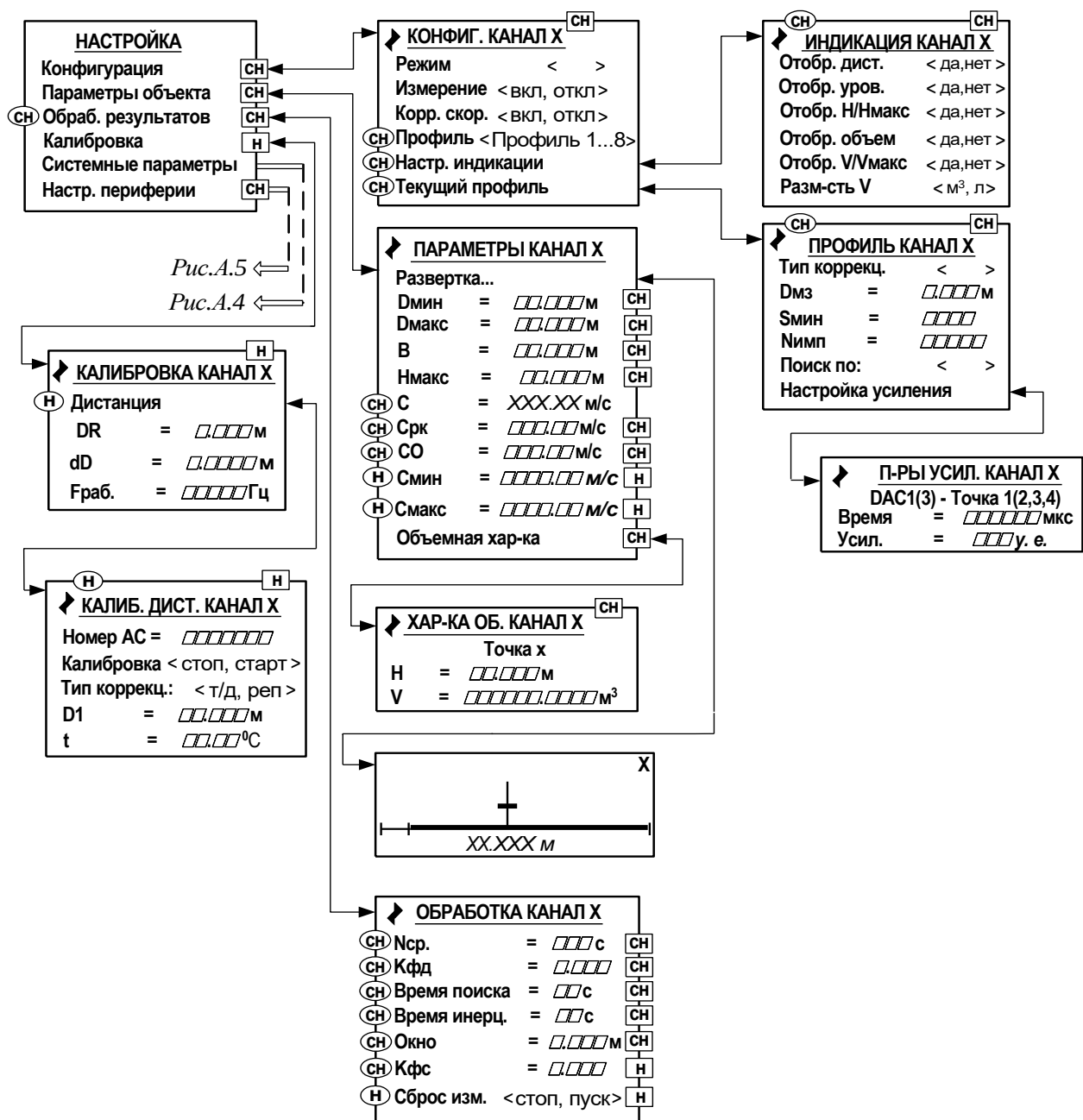
Рис.А.3. Меню «Настройка», «Конфигурация», «Параметры объекта», «Обработка результатов» и «Калибровка».
