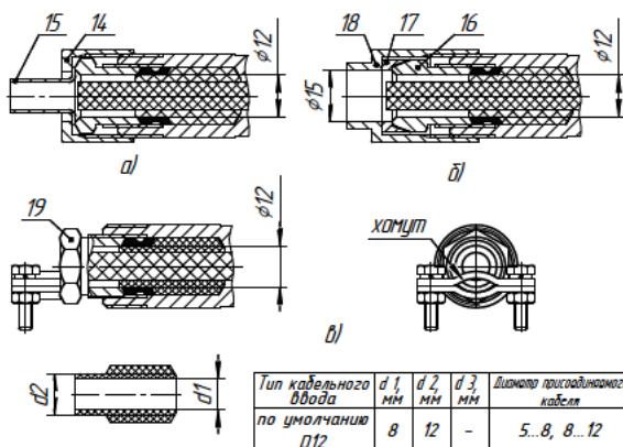
Рис. А.3 - Внешний вид БПК-12(24)В-2Р-ГС-В31. Чертеж средств взрывозащиты
