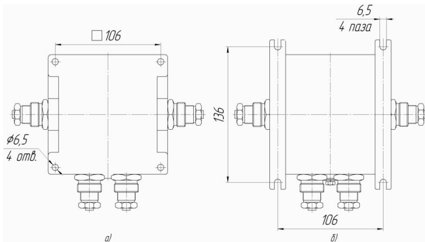
Рис.А.5 – Посадочные места БПК. а) без крепежных пластин; б) с крепежными пластинами.
