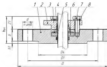
1 - фланец; 2 - вкладыш; 3 - шайба; 4 - цапга; 5 - кольцо уплотнительное; 6 - прокладка; 7 - болт; 8 - шайба пружинная.
