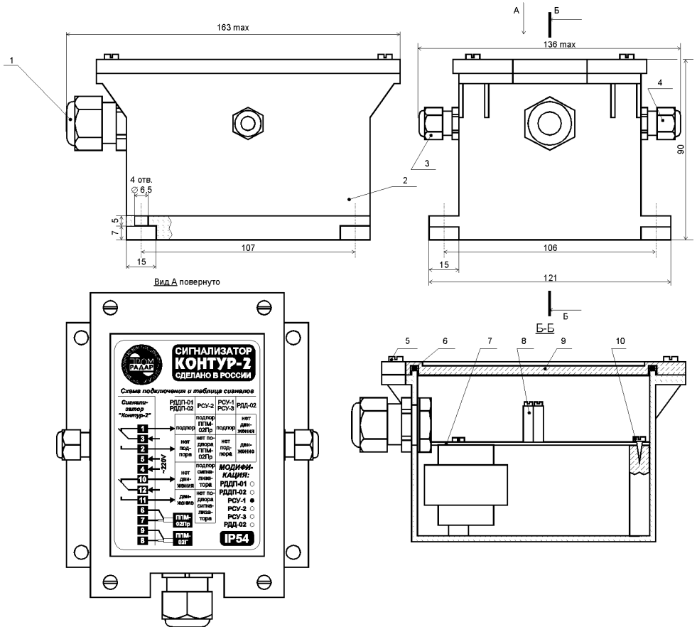
Рис. 1. Конструкция сигнализатора «Контур-2» (модификация «PCY-1»).
