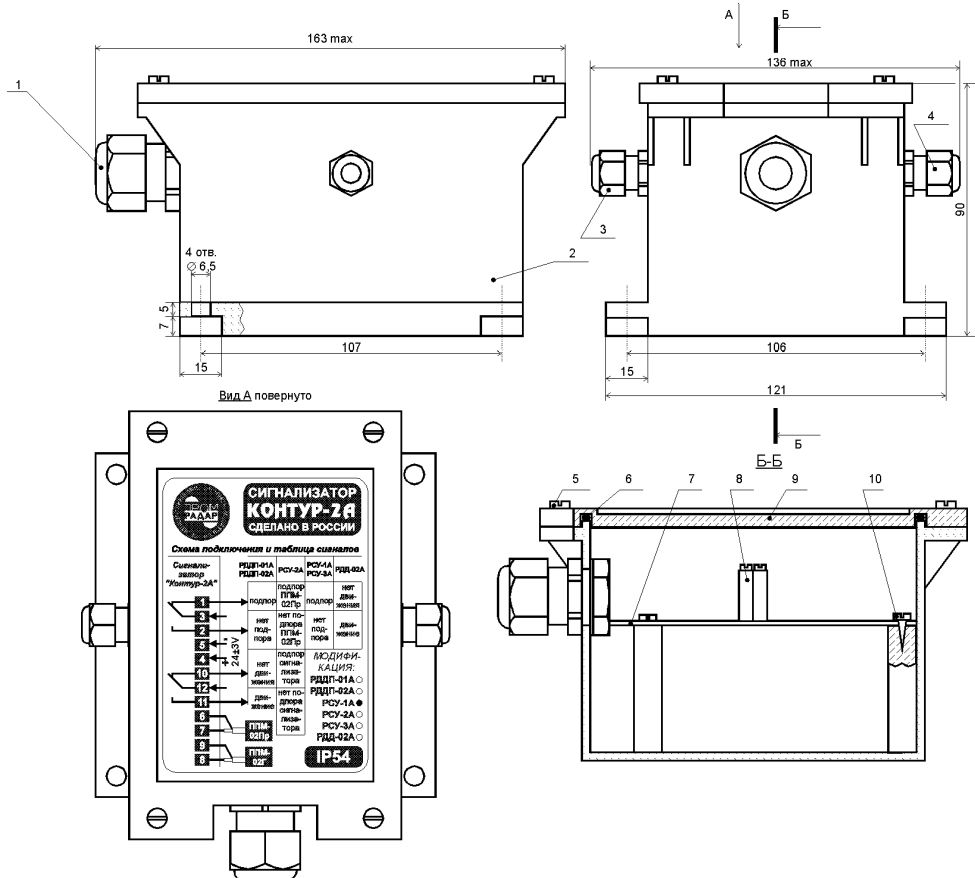
Рис. 4. Конструкция сигнализатора «Контур-2А» (модификация «PCY-1A»).
