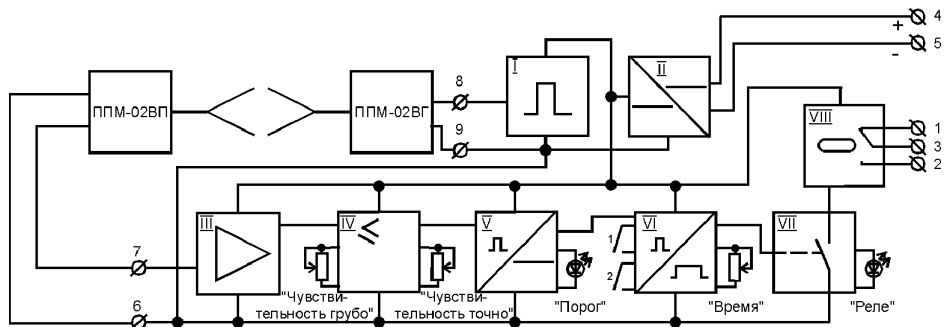
Рис. 2. Структурная схема датчика PCSU-1P-2A.
