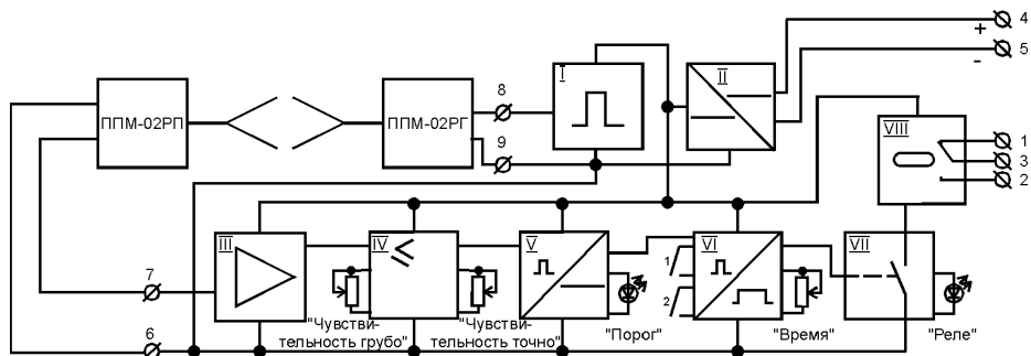
Рис. 2. Структурная схема датчика РСУ-1РА.
