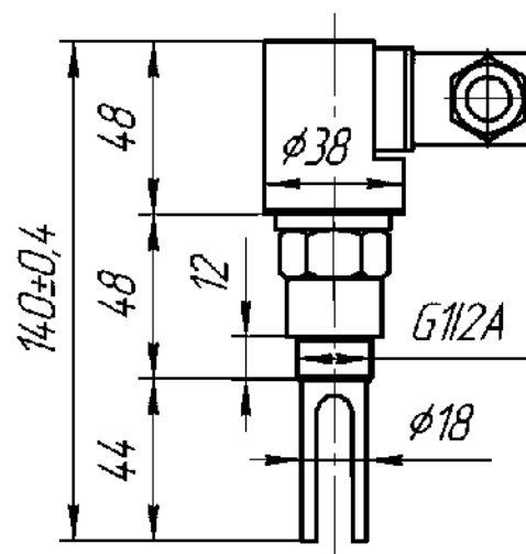
СКАТ-5М-К-Б(1/2)
