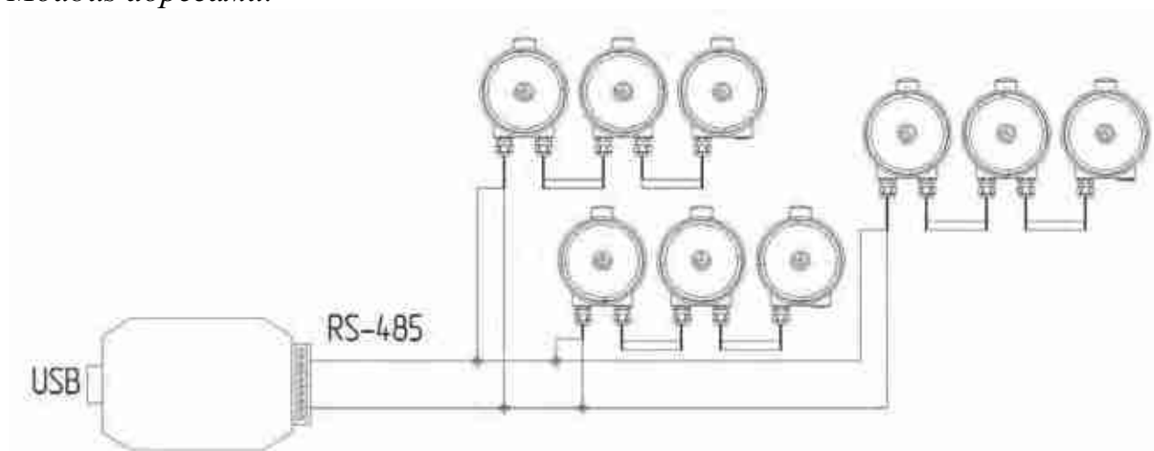
Рис. 6.5 Способ прокладки линии RS-485 «звезда»
