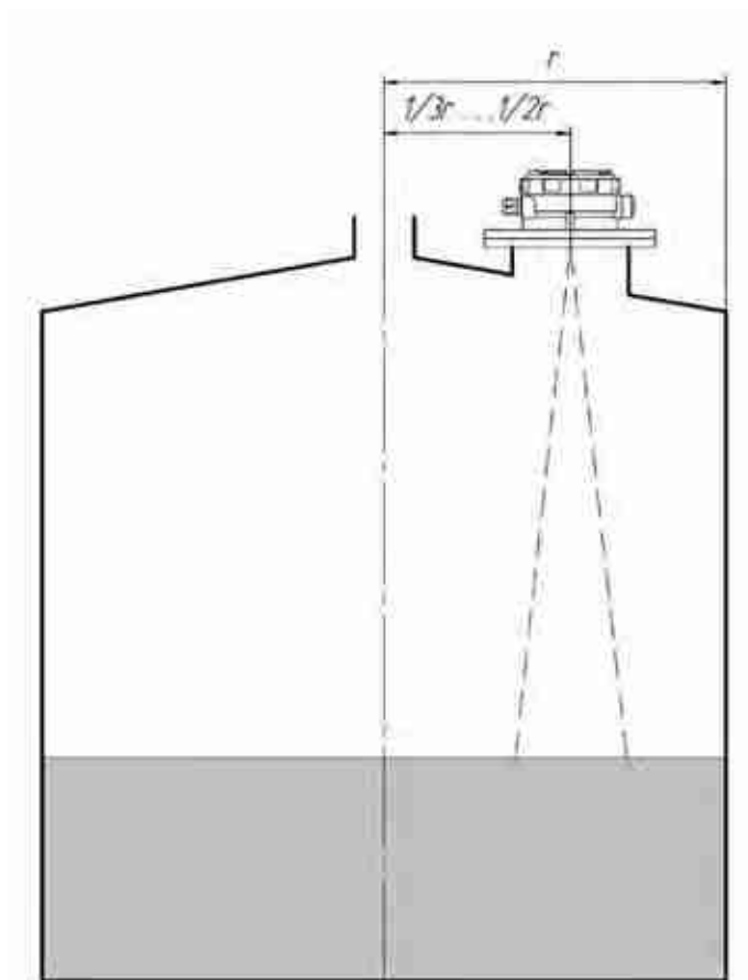
Рис. 4.7. Установка прибора
