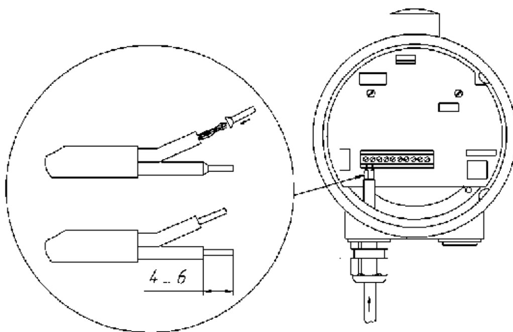
Рис. 4.20 Подключение датчика
