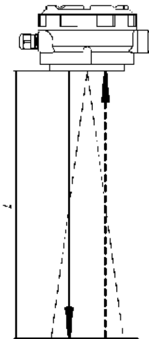
Рис. 3.5. Принцип измерения.
