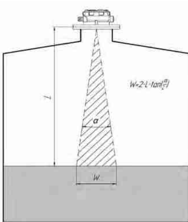
Рис. 4.10. Зона действия измерительного луча
