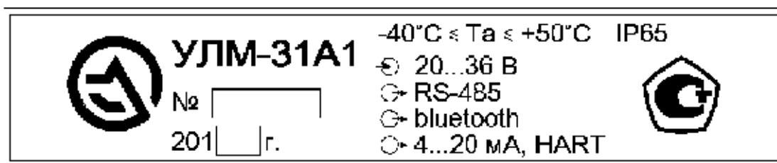
Рис. 3.3. Типовой шильдик
